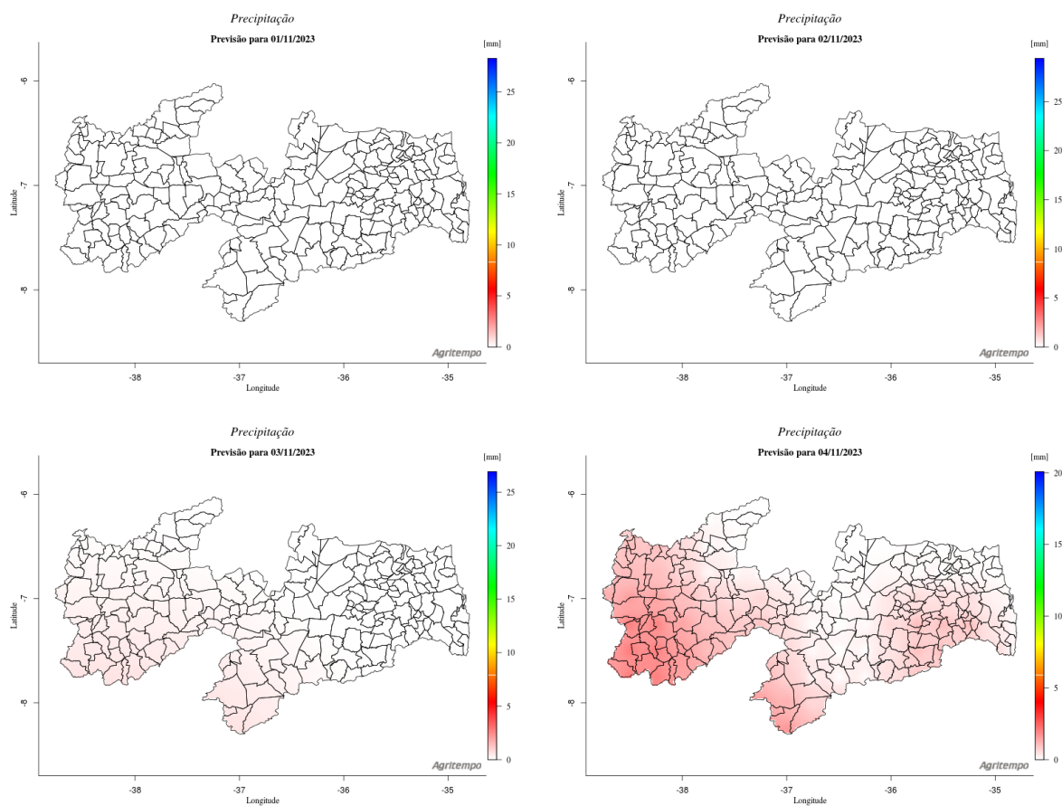
Figura 3 - Previsão de precipitação para a Paraíba nos dias 01 a 04 de novembro de 2023. Agritempo/Embrapa.
