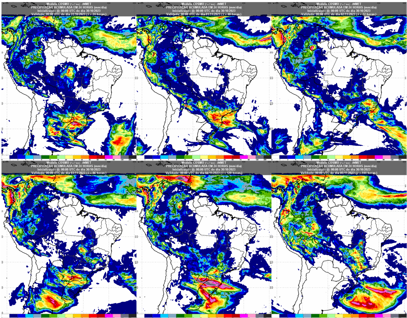
Figura 2 – Previsão de precipitação para o Brasil nos dias 31 de outubro a 05 de novembro de 2023. INMET
