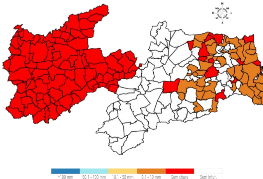
Figura 1 - Acumulado de precipitação nos municípios da Paraíba entre 23 a 29 de outubro. AESA
