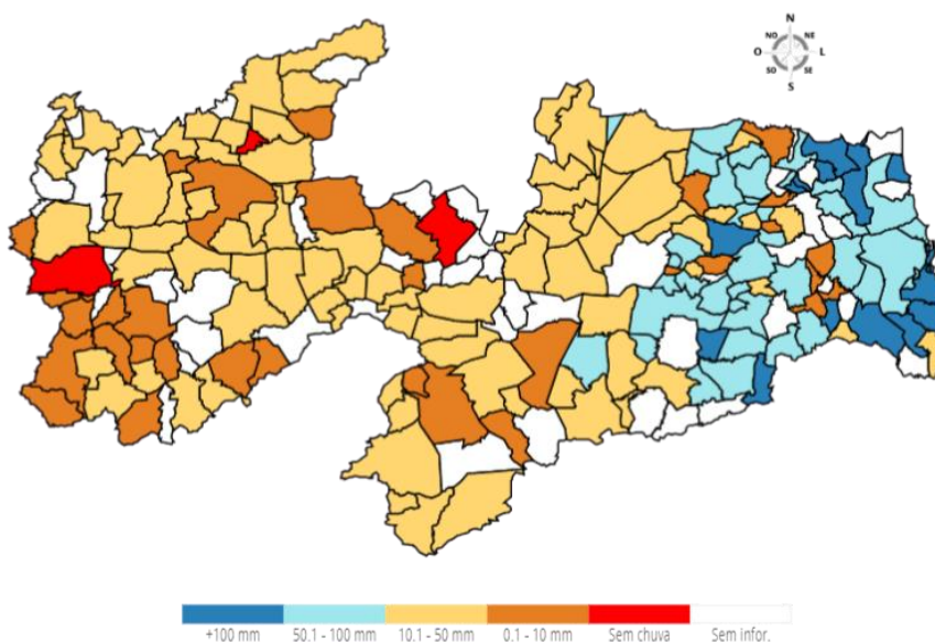
Figura 1 - Acumulado de precipitação nos municípios da Paraíba entre 10 a 16 de junho de 2024. AESA
