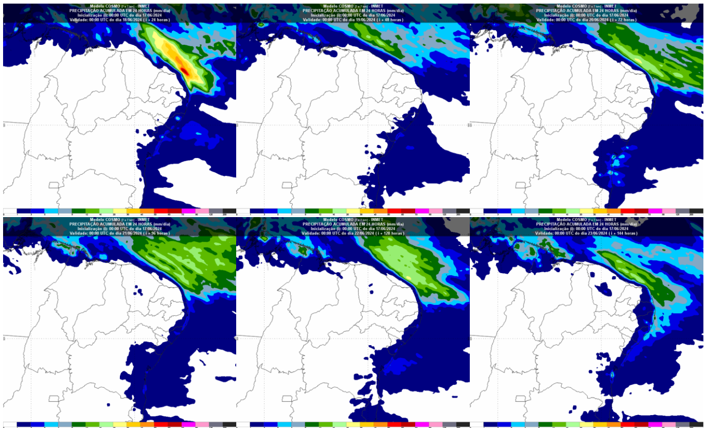
Figura 2 – Previsão de precipitação para o Nordeste nos dias 18 a 23 de junho de 2024. INMET
